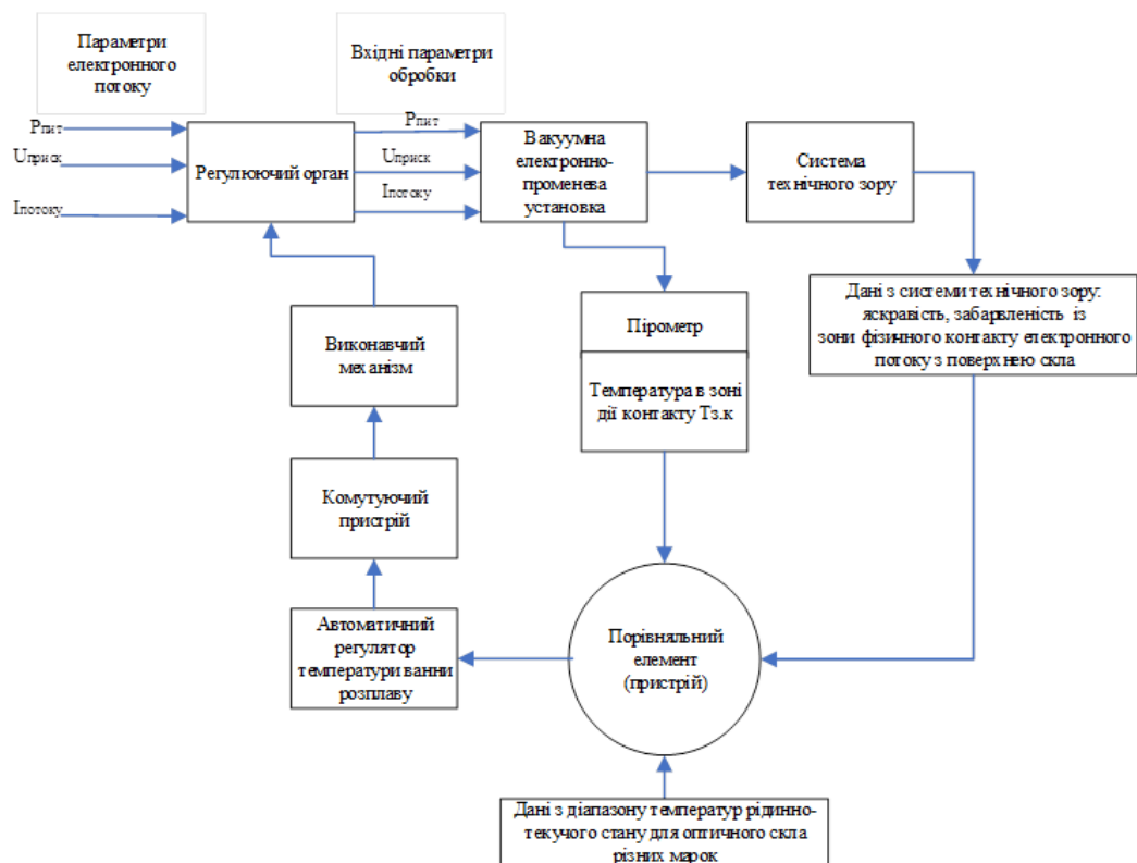
Рис. 2. Структурна схема системи спостереження та автоматичного контролю і регулювання температури на поверхні ванни розплаву з використанням технічного зору і пірометра
