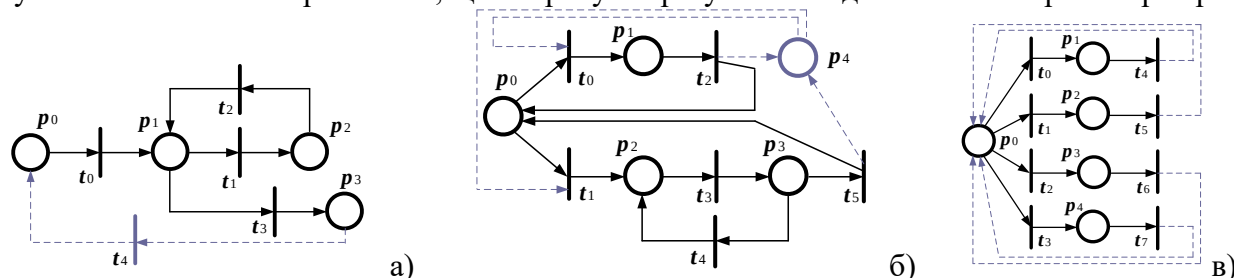
Рис. 1. Фрагменти PN-моделі: а – з одиничними входом та виходом, б – з двома входами та виходами; в – з множинними входами та виходами
