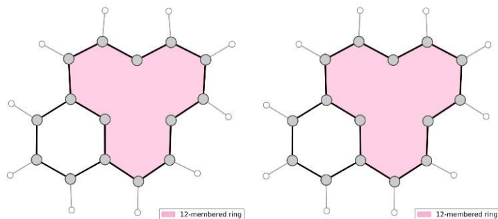
Рис. 1. Центральна моновакансія пірену: DFT (ліворуч, \Delta E_f = 8.06 eB) та MLIP (праворуч, \Delta E_f = 7.08 eB). Обидва методи дають 5–9 ян-теллерівську реконструкцію (синім – пентагон, фіолетовим – нонагон) з ненасиченим радикалом і локальним магнітним [2]
