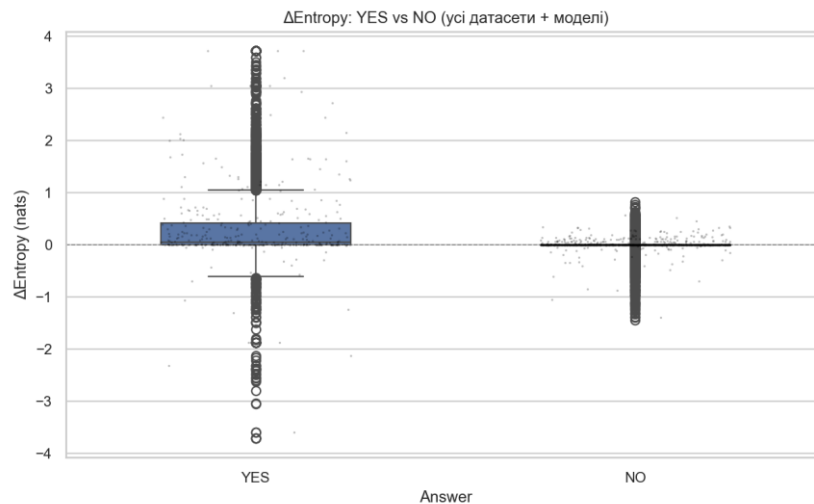
Рис. 1. Розподіли \Delta Entropy для відповідей YES та NO (36 000 крок-замірів, всі датасети та моделі). Шкала логарифмічна за віссю Y
