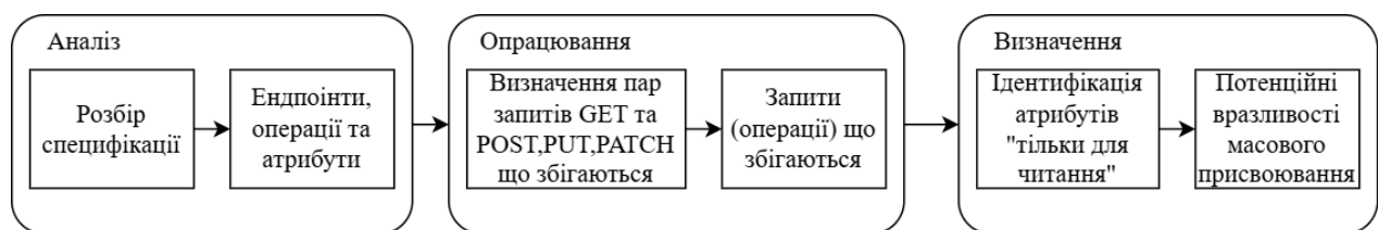
Рис. 1. Схеми визначення вразливості масового присвоювання
