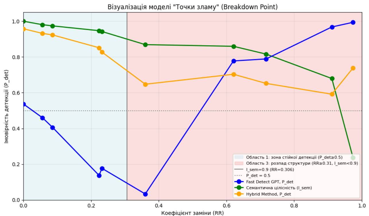
Рис. 1. Модель Точки зламу для гібридного методу детекції
