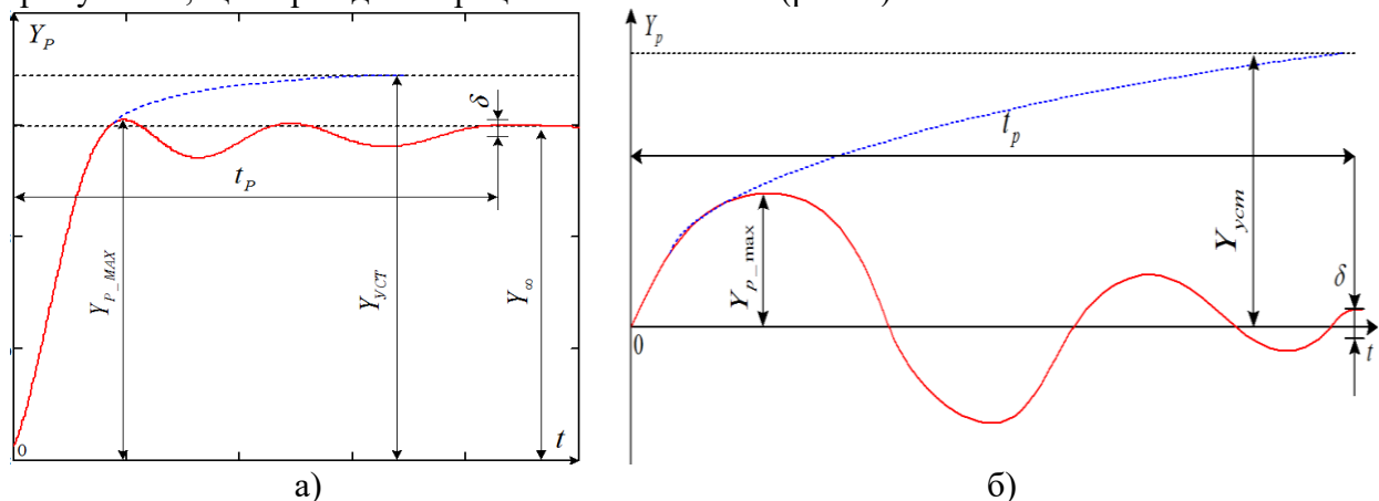
Рис. 1. Типові перехідні процеси у системах: а) – астатичній; б) – статичній
