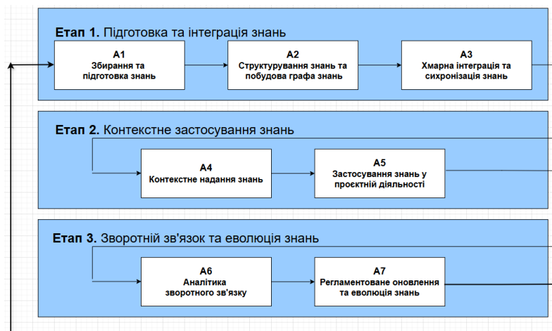
Рис. 1. Функціональна декомпозиція процесної моделі CIKML (A1-A7)
