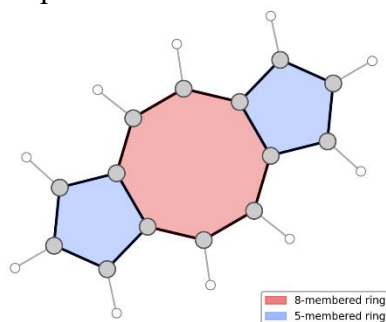
Рис. 3. Центральна дивакансія пірену дає канонічну реконструкцію 5–8–5 (синім – пентагони, червоним – октагон)
