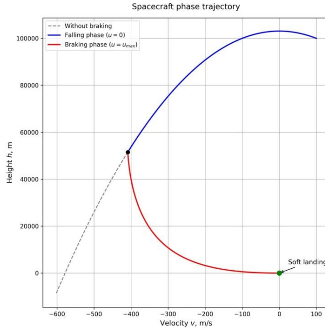
Fig. 1. Phase Trajectory
