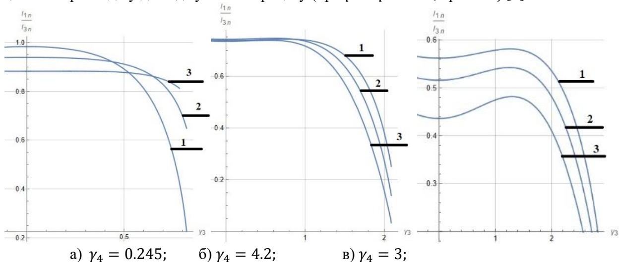
Рис. 1. Залежність кількості добутої інформації I_{1n}/I_{3n} з вибіркових значень про розрізнення гіпотез від коефіцієнта асиметрії при використанні поліноміальних РП при асиметрично-ексцесній заваді при різних значеннях коефіцієнта ексцесу \gamma_4 та відношенні сигнал/завада 1) p_1 = p_2 = 1 ; 2) p_1 = p_2 = 0.5 ; 3) p_1 = p_2 = 0.1
