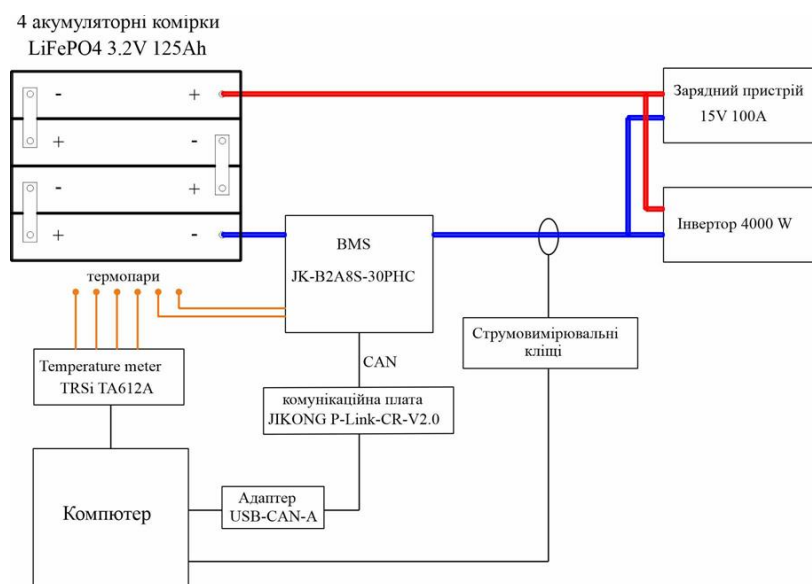
Рис. 1. Структурна схема експериментальної установки та системи збору даних для акумуляторного модуля, включаючи канали електричних та теплових вимірювань
