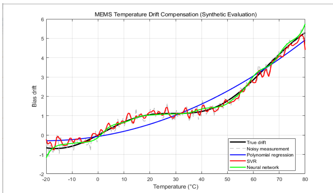
Рис. 1. Моделювання температурно-залежного дрейфу зміщення MEMS-сенсора та порівняння методів компенсації на основі поліноміальної регресії, регресії опорних векторів та нейромережевих моделей
