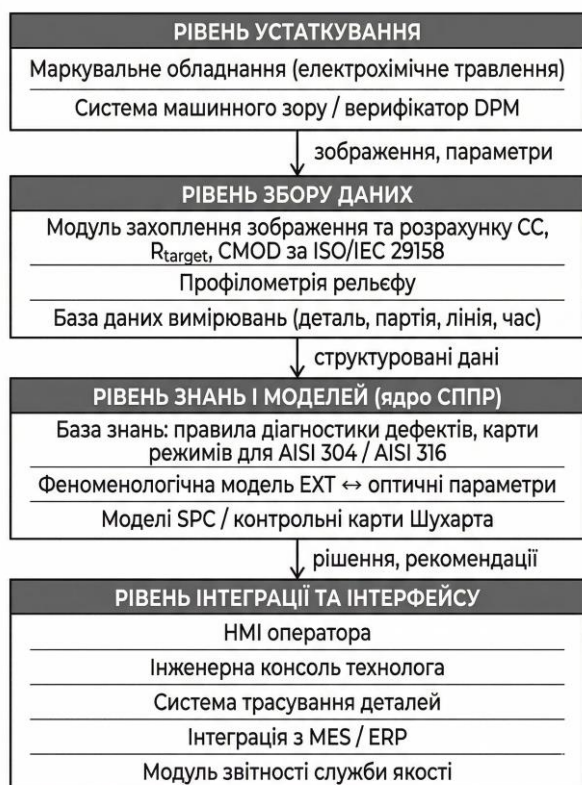
Рис. 1. а) Концептуальна схема СППР контролю якості DPM-маркування б) Алгоритм прийняття рішень СППР
