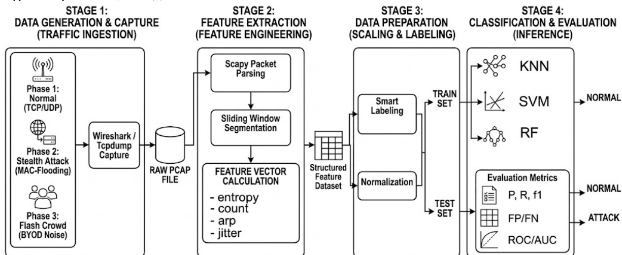
Рис. 1. Конвеєр обробки даних для виявлення MAC-Flooding
