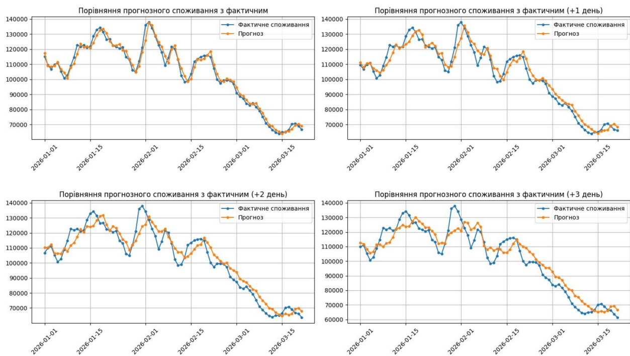
Рис. 2. Співставлення фактичних і модельних даних в залежності від широти горизонту прогнозування для України загалом
