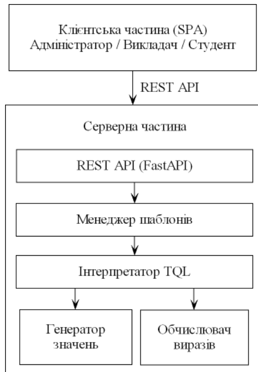
Рис. 1. Структура інформаційної системи
