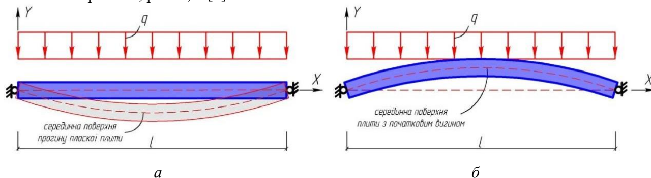
Рис. 1. Схема шарнірно обпертої плити: а – плоска плита; б – плита з початковим вигином
