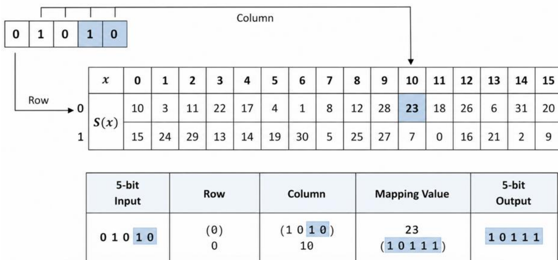
Рис. 1. Структура 5-бітного S-блоку
