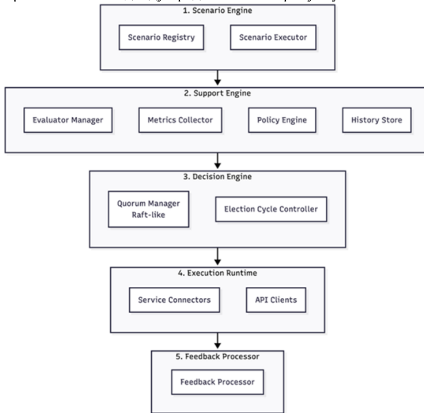
Рис. 1. Архітектура SDRS
