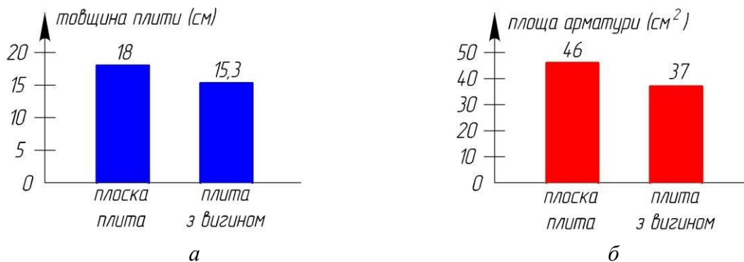
Рис. 2. Діаграми зменшення товщини (а) та кількості арматури (б) плити перекриття з початковим вигином у порівнянні з плоскою плитою
