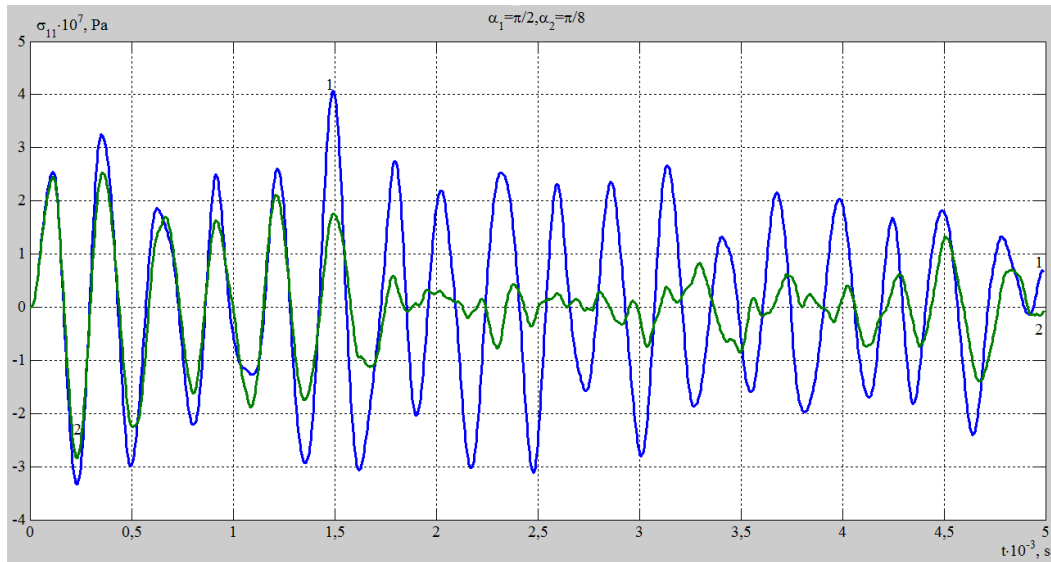
Рис. 1. Залежність величини напруження \sigma_{11} від часу t в точці \alpha_1 = \frac{\pi}{2}, \alpha_2 = \frac{\pi}{8}
