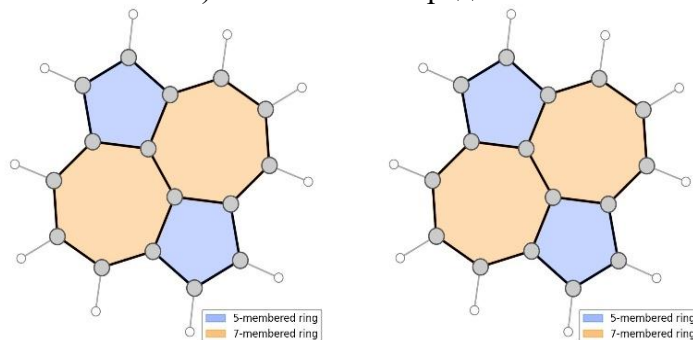
Рис. 2. Центральний дефект Стоуна–Уельса пірену: DFT (ліворуч, \Delta E_f = 1.96 eB) та MLIP (праворуч, \Delta E_f = 2.01 eB). Обидва методи дають канонічну топологію 5–7–7–5 (синім – пентагони, помаранчевим – гептагони) [5]
