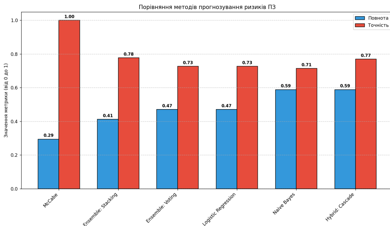
Рис. 1. Порівняння індивідуальних та ансамблевих методів прогнозування ризиків ПЗ
