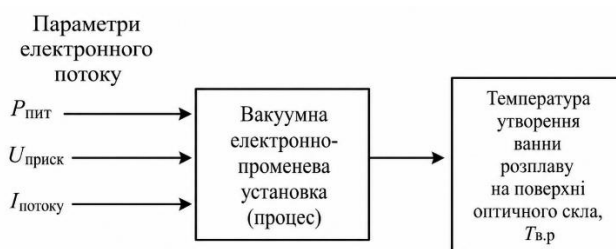
Рис. 1. Схема процесу електронно-променевої обробки поверхні оптичного скла з утворенням ванни розплаву
