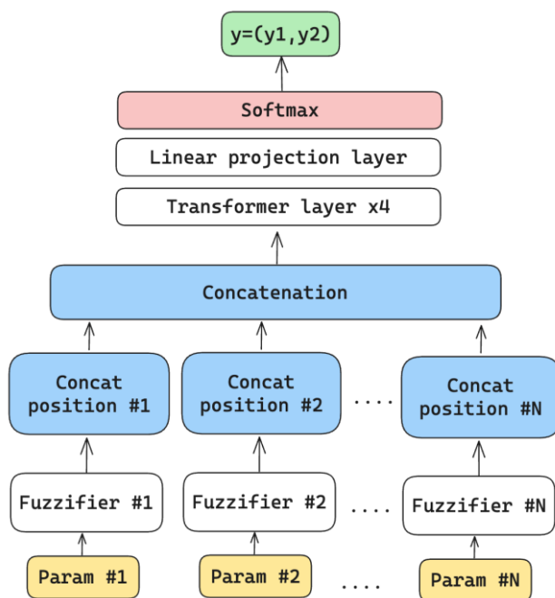
Рис. 1. Архітектура нейронної мережі FTNNB
