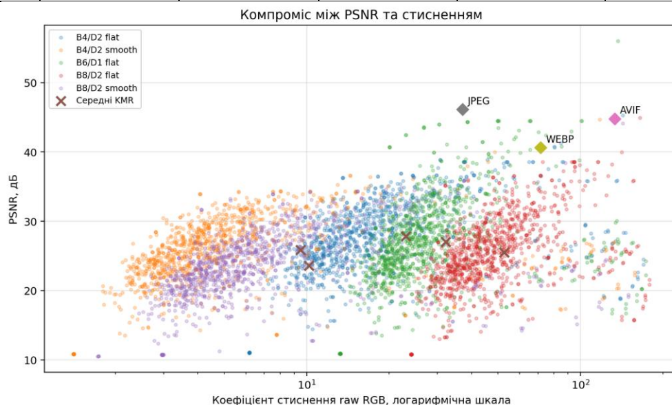
Рис. 1. Компроміс між PSNR і коефіцієнтом стиснення
